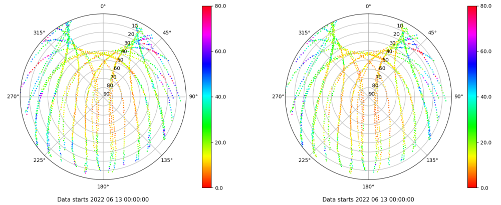
Skyplot for station LPAL. Parameter M1C Data file LPAL00ESP_R_2022164.xtr Skyplot for station LPAL. Parameter M2C Data file LPAL00ESP_R_2022164.xtr
