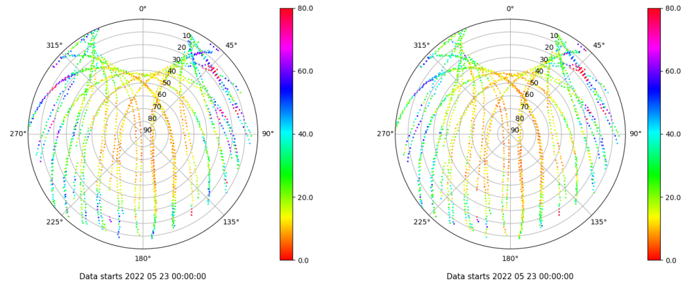
Skyplot for station LPAL. Parameter M1C Data file LPAL00ESP_R_2022143.xtr Skyplot for station LPAL. Parameter M2C Data file LPAL00ESP_R_2022143.xtr
