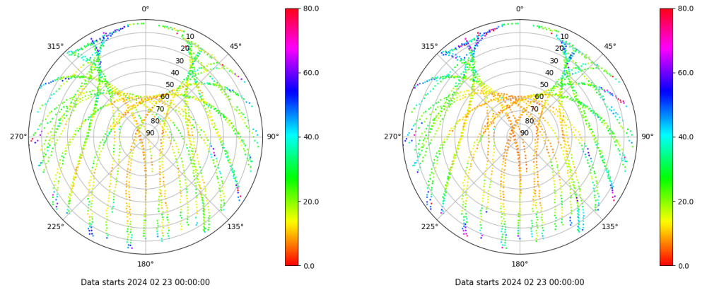
Skyplot for station JACA. Parameter M1C Data file JACA00ESP_R_2024054.xtr Skyplot for station JACA. Parameter M2P Data file JACA00ESP_R_2024054.xtr
