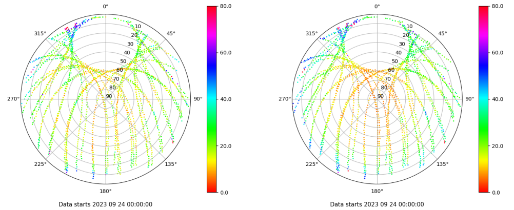
Skyplot for station JACA. Parameter M1C Data file JACA00ESP_R_2023267.xtr Skyplot for station JACA. Parameter M2P Data file JACA00ESP_R_2023267.xtr
