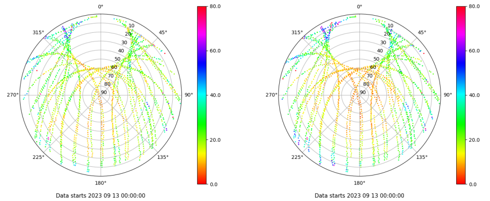
Skyplot for station JACA. Parameter M1C Data file JACA00ESP_R_2023256.xtr Skyplot for station JACA. Parameter M2P Data file JACA00ESP_R_2023256.xtr
