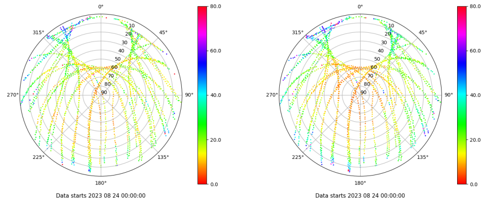
Skyplot for station JACA. Parameter M1C Data file JACA00ESP_R_2023236.xtr Skyplot for station JACA. Parameter M2P Data file JACA00ESP_R_2023236.xtr
