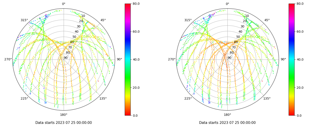
Skyplot for station JACA. Parameter M1C Data file JACA00ESP_R_2023206.xtr Skyplot for station JACA. Parameter M2P Data file JACA00ESP_R_2023206.xtr
