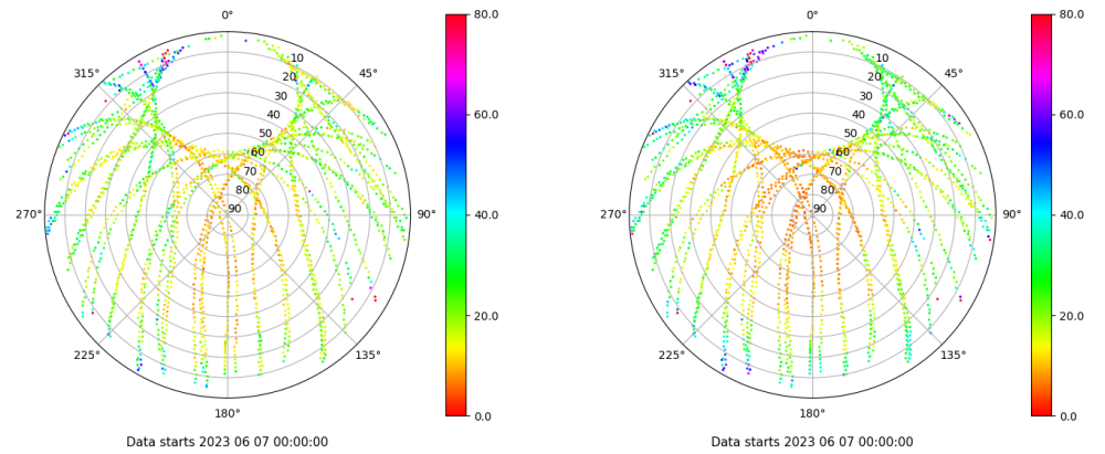
Skyplot for station JACA. Parameter M1C Data file JACA00ESP_R_2023158.xtr Skyplot for station JACA. Parameter M2P Data file JACA00ESP_R_2023158.xtr
