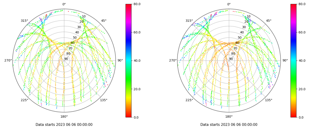
Skyplot for station JACA. Parameter M1C Data file JACA00ESP_R_2023157.xtr Skyplot for station JACA. Parameter M2P Data file JACA00ESP_R_2023157.xtr
