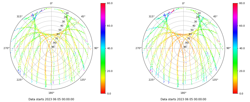
Skyplot for station JACA. Parameter M1C Data file JACA00ESP_R_2023156.xtr Skyplot for station JACA. Parameter M2P Data file JACA00ESP_R_2023156.xtr
