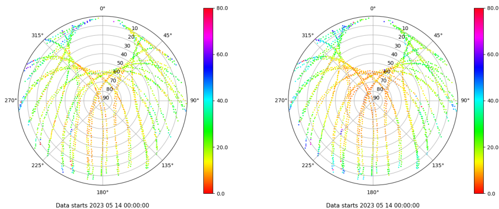
Skyplot for station JACA. Parameter M1C Data file JACA00ESP_R_2023134.xtr Skyplot for station JACA. Parameter M2P Data file JACA00ESP_R_2023134.xtr
