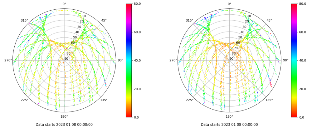
Skyplot for station JACA. Parameter M1C Data file JACA00ESP_R_2023008.xtr Skyplot for station JACA. Parameter M2P Data file JACA00ESP_R_2023008.xtr
