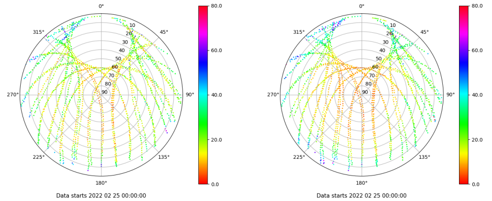
Skyplot for station JACA. Parameter M1C Data file JACA00ESP_R_2022056.xtr Skyplot for station JACA. Parameter M2P Data file JACA00ESP_R_2022056.xtr
