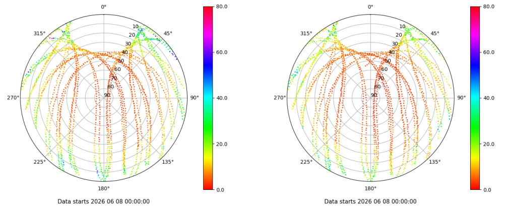
Skyplot for station IZAN. Parameter M1C Data file IZAN00ESP_R_2026159.xtr Skyplot for station IZAN. Parameter M2C Data file IZAN00ESP_R_2026159.xtr
