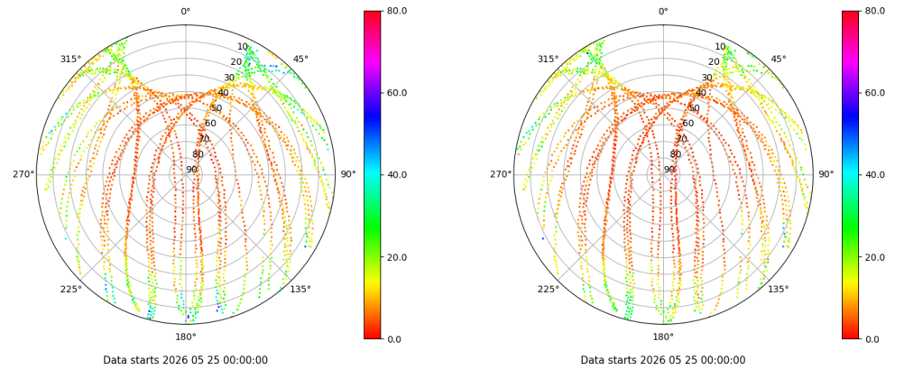
Skyplot for station IZAN. Parameter M1C Data file IZAN00ESP_R_2026145.xtr Skyplot for station IZAN. Parameter M2C Data file IZAN00ESP_R_2026145.xtr
