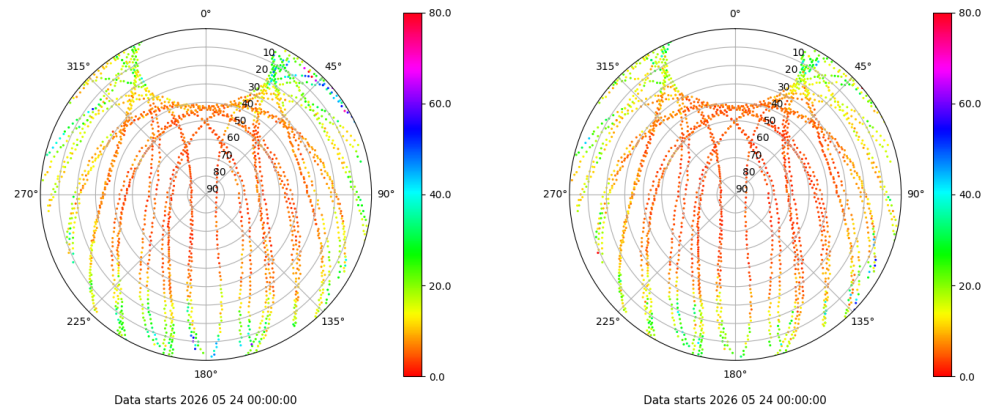
Skyplot for station IZAN. Parameter M1C Data file IZAN00ESP_R_2026144.xtr Skyplot for station IZAN. Parameter M2C Data file IZAN00ESP_R_2026144.xtr
