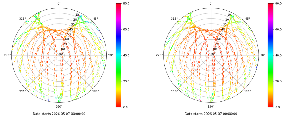
Skyplot for station IZAN. Parameter M1C Data file IZAN00ESP_R_2026127.xtr Skyplot for station IZAN. Parameter M2C Data file IZAN00ESP_R_2026127.xtr
