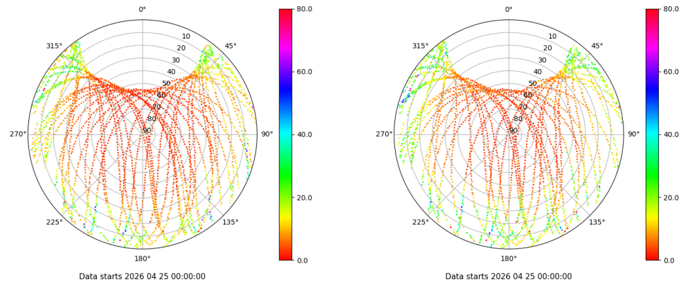
Skyplot for station IZAN. Parameter M1C Data file IZAN00ESP_R_2026115.xtr Skyplot for station IZAN. Parameter M2S Data file IZAN00ESP_R_2026115.xtr
