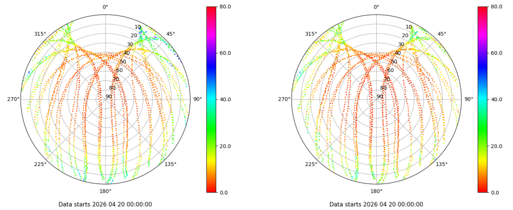
Skyplot for station IZAN. Parameter M1C Data file IZAN00ESP_R_2026110.xtr Skyplot for station IZAN. Parameter M2C Data file IZAN00ESP_R_2026110.xtr
