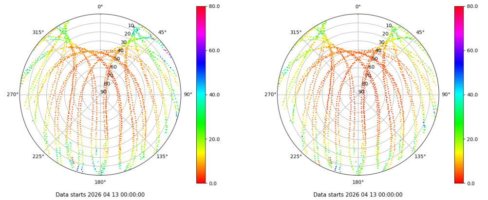
Skyplot for station IZAN. Parameter M1C Data file IZAN00ESP_R_2026103.xtr Skyplot for station IZAN. Parameter M2C Data file IZAN00ESP_R_2026103.xtr
