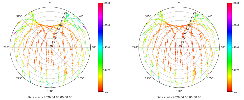
Skyplot for station IZAN. Parameter M1C Data file IZAN00ESP_R_2026096.xtr Skyplot for station IZAN. Parameter M2C Data file IZAN00ESP_R_2026096.xtr
