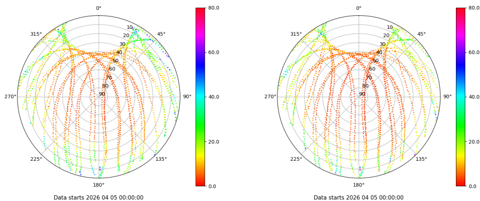
Skyplot for station IZAN. Parameter M1C Data file IZAN00ESP_R_2026095.xtr Skyplot for station IZAN. Parameter M2C Data file IZAN00ESP_R_2026095.xtr
