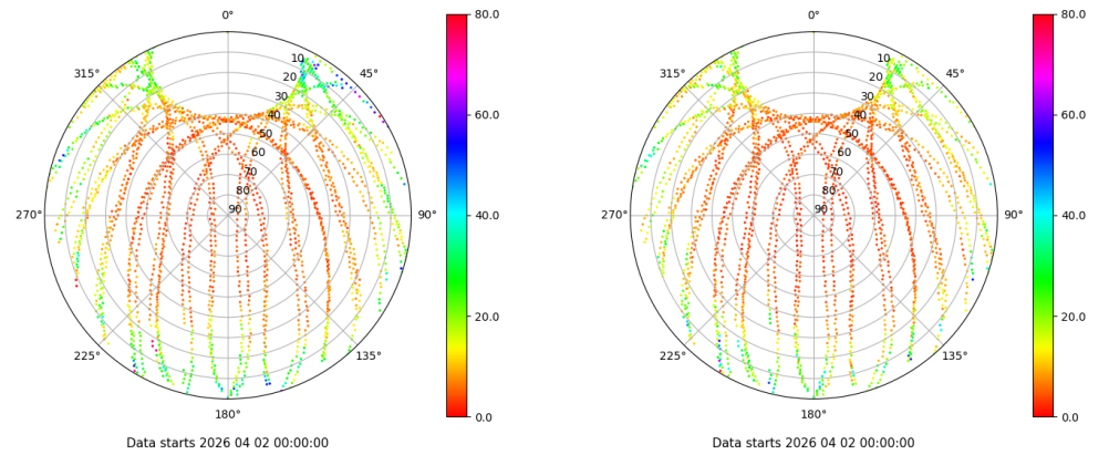
Skyplot for station IZAN. Parameter M1C Data file IZAN00ESP_R_2026092.xtr Skyplot for station IZAN. Parameter M2C Data file IZAN00ESP_R_2026092.xtr
