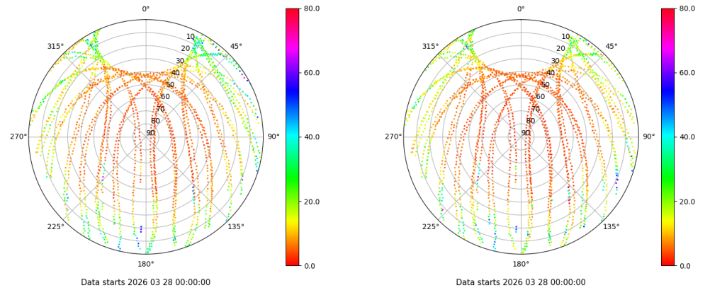
Skyplot for station IZAN. Parameter M1C Data file IZAN00ESP_R_2026087.xtr Skyplot for station IZAN. Parameter M2C Data file IZAN00ESP_R_2026087.xtr
