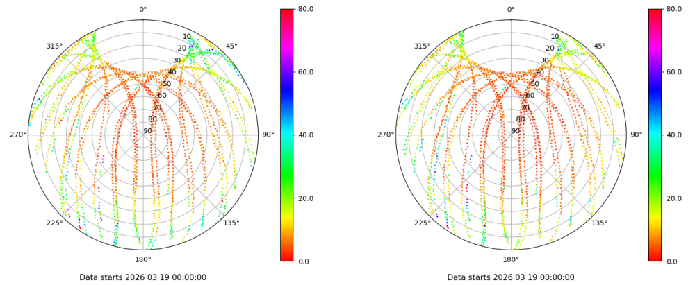
Skyplot for station IZAN. Parameter M1C Data file IZAN00ESP_R_2026078.xtr Skyplot for station IZAN. Parameter M2C Data file IZAN00ESP_R_2026078.xtr
