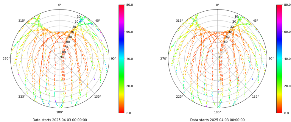
Skyplot for station IZAN. Parameter M1C Data file IZAN00ESP_R_2025093.xtr Skyplot for station IZAN. Parameter M2C Data file IZAN00ESP_R_2025093.xtr
