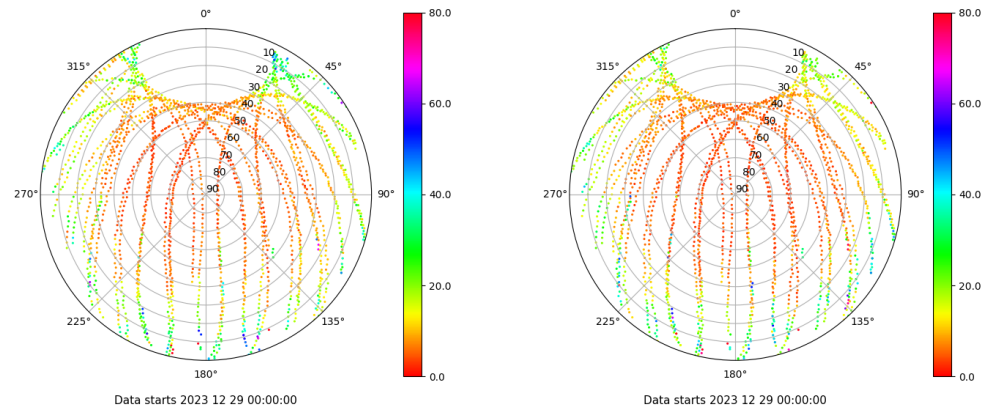
Skyplot for station IZAN. Parameter M1C Data file IZAN00ESP_R_2023363.xtr Skyplot for station IZAN. Parameter M2C Data file IZAN00ESP_R_2023363.xtr
