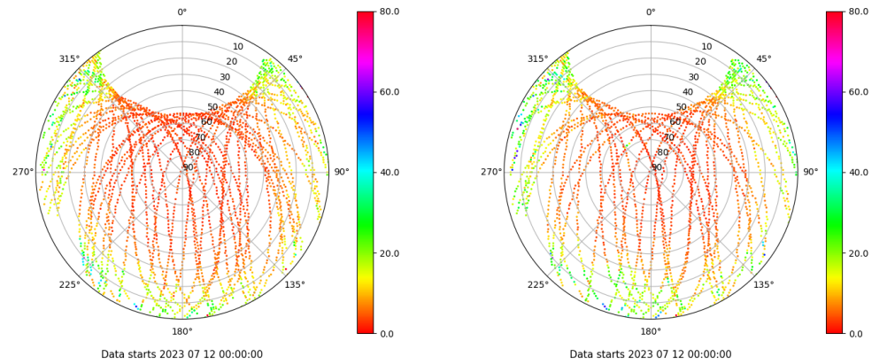
Skyplot for station IZAN. Parameter M1C Data file IZAN00ESP_R_2023193.xtr Skyplot for station IZAN. Parameter M2S Data file IZAN00ESP_R_2023193.xtr
