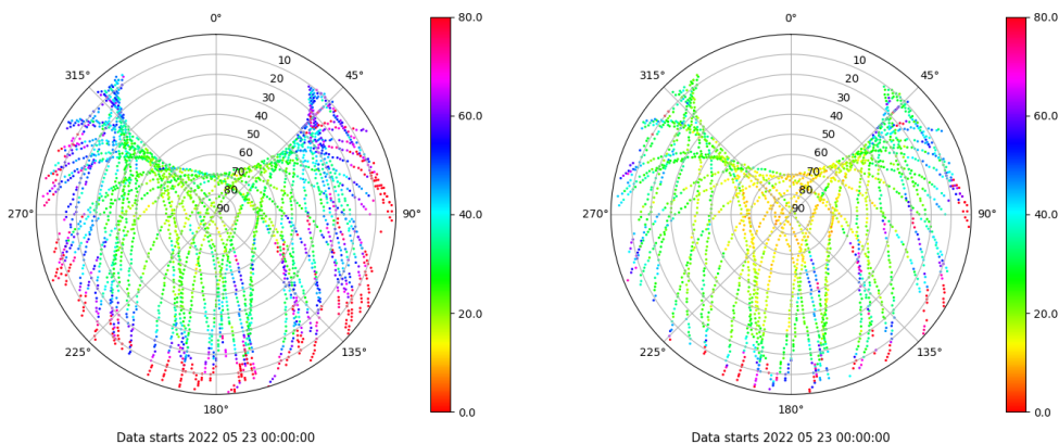
Skyplot for station ICOL. Parameter M1C Data file ICOL00ESP_R_2022143.xtr Skyplot for station ICOL. Parameter M2X Data file ICOL00ESP_R_2022143.xtr
