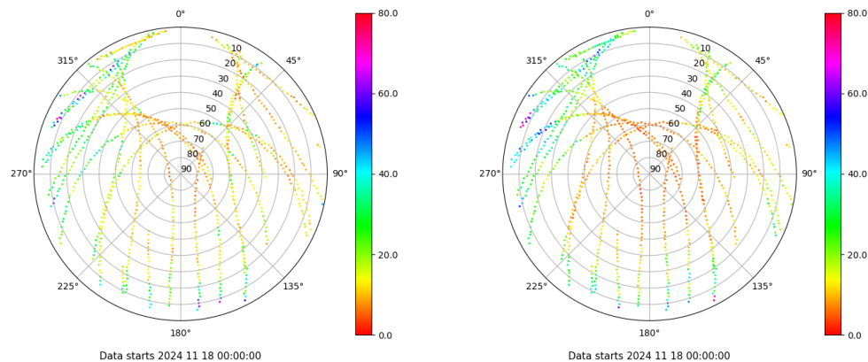
Skyplot for station GIRO. Parameter M1C Data file GIRO00ESP_R_2024323.xtr Skyplot for station GIRO. Parameter M2P Data file GIRO00ESP_R_2024323.xtr
