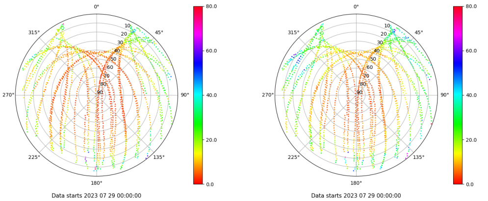
Skyplot for station FUER. Parameter M1C Data file FUER00ESP_R_2023210.xtr Skyplot for station FUER. Parameter M2P Data file FUER00ESP_R_2023210.xtr
