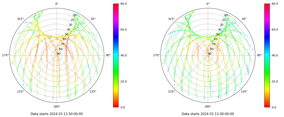
Skyplot for station CAZA. Parameter M1C Data file CAZA00ESP_R_2024073.xtr Skyplot for station CAZA. Parameter M2P Data file CAZA00ESP_R_2024073.xtr
