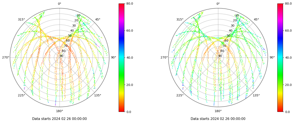
Skyplot for station CAZA. Parameter M1C Data file CAZA00ESP_R_2024057.xtr Skyplot for station CAZA. Parameter M2P Data file CAZA00ESP_R_2024057.xtr
