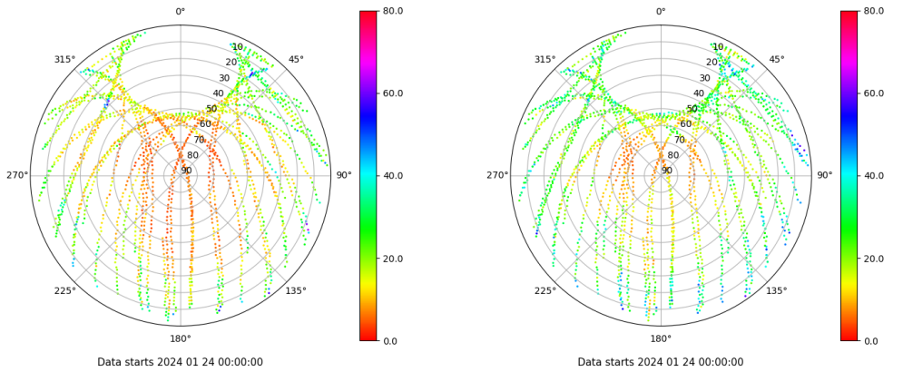
Skyplot for station CAZA. Parameter M1C Data file CAZA00ESP_R_2024024.xtr Skyplot for station CAZA. Parameter M2P Data file CAZA00ESP_R_2024024.xtr
