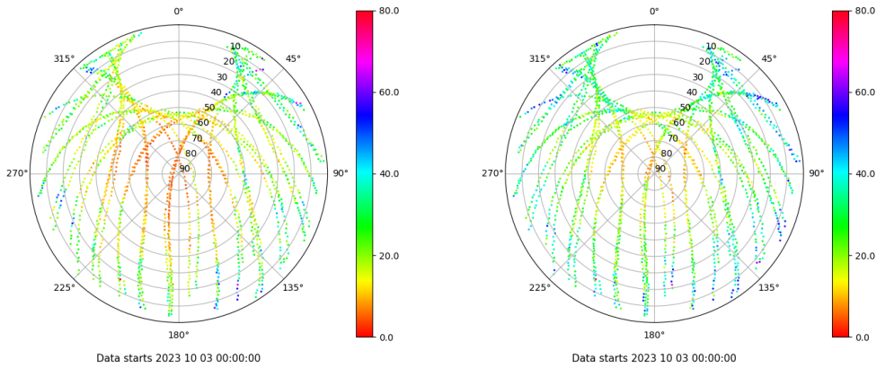
Skyplot for station CAZA. Parameter M1C Data file CAZA00ESP_R_2023276.xtr Skyplot for station CAZA. Parameter M2P Data file CAZA00ESP_R_2023276.xtr
