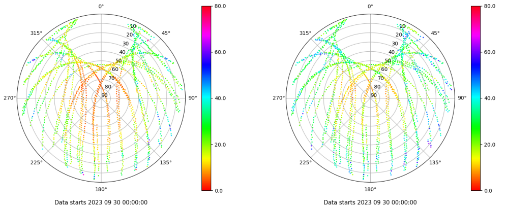
Skyplot for station CAZA. Parameter M1C Data file CAZA00ESP_R_2023273.xtr Skyplot for station CAZA. Parameter M2P Data file CAZA00ESP_R_2023273.xtr
