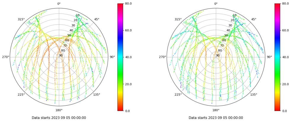
Skyplot for station CAZA. Parameter M1C Data file CAZA00ESP_R_2023248.xtr Skyplot for station CAZA. Parameter M2P Data file CAZA00ESP_R_2023248.xtr
