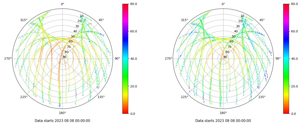
Skyplot for station CAZA. Parameter M1C Data file CAZA00ESP_R_2023220.xtr Skyplot for station CAZA. Parameter M2P Data file CAZA00ESP_R_2023220.xtr
