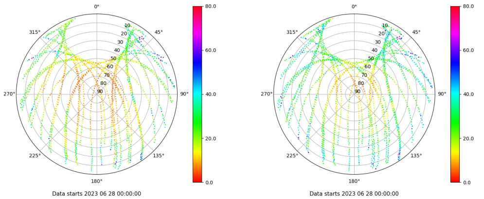
Skyplot for station CAZA. Parameter M1C Data file CAZA00ESP_R_2023179.xtr Skyplot for station CAZA. Parameter M2P Data file CAZA00ESP_R_2023179.xtr
