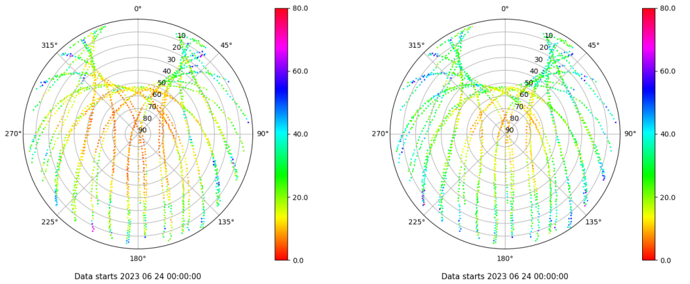
Skyplot for station CAZA. Parameter M1C Data file CAZA00ESP_R_2023175.xtr Skyplot for station CAZA. Parameter M2P Data file CAZA00ESP_R_2023175.xtr
