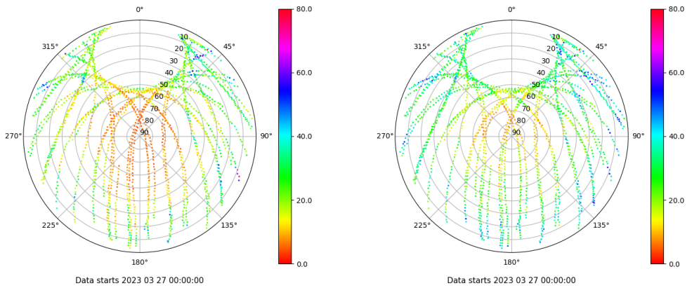
Skyplot for station CAZA. Parameter M1C Data file CAZA00ESP_R_2023086.xtr Skyplot for station CAZA. Parameter M2P Data file CAZA00ESP_R_2023086.xtr
