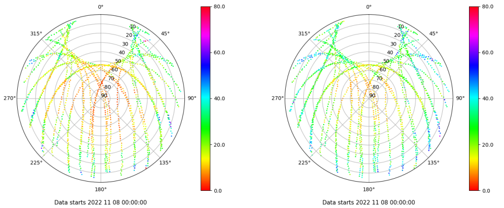
Skyplot for station CAZA. Parameter M1C Data file CAZA00ESP_R_2022312.xtr Skyplot for station CAZA. Parameter M2P Data file CAZA00ESP_R_2022312.xtr
