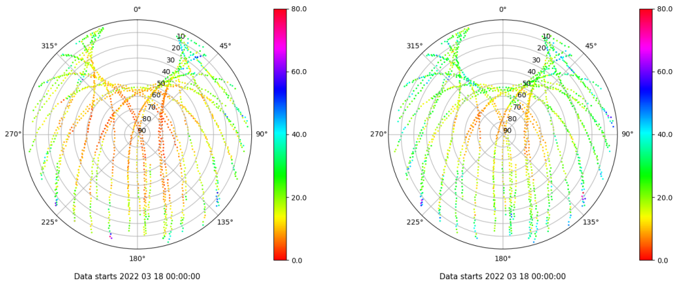
Skyplot for station CAZA. Parameter M1C Data file CAZA00ESP_R_2022077.xtr Skyplot for station CAZA. Parameter M2P Data file CAZA00ESP_R_2022077.xtr
