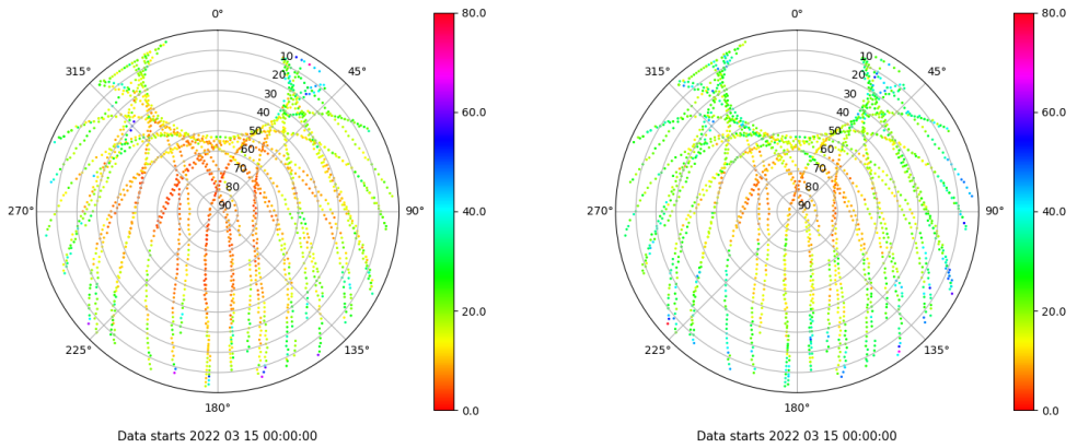
Skyplot for station CAZA. Parameter M1C Data file CAZA00ESP_R_2022074.xtr Skyplot for station CAZA. Parameter M2P Data file CAZA00ESP_R_2022074.xtr
