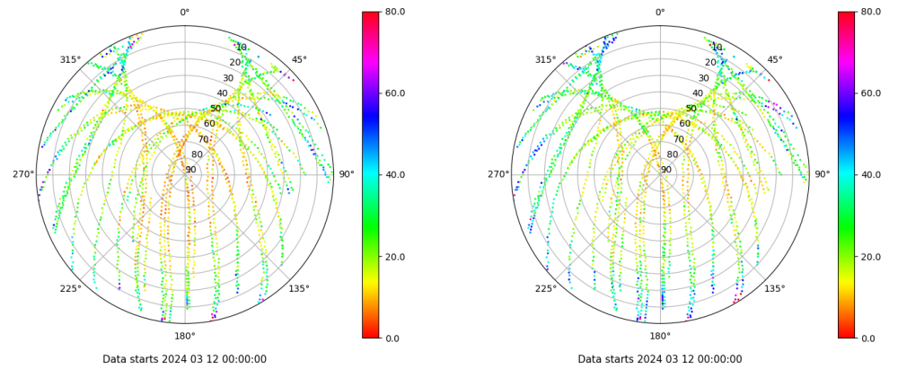
Skyplot for station CAAL. Parameter M1C Data file CAAL00ESP_R_2024072.xtr Skyplot for station CAAL. Parameter M2P Data file CAAL00ESP_R_2024072.xtr
