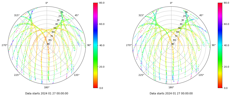
Skyplot for station CAAL. Parameter M1C Data file CAAL00ESP_R_2024027.xtr Skyplot for station CAAL. Parameter M2P Data file CAAL00ESP_R_2024027.xtr
