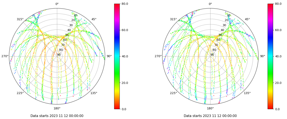
Skyplot for station CAAL. Parameter M1C Data file CAAL00ESP_R_2023316.xtr Skyplot for station CAAL. Parameter M2P Data file CAAL00ESP_R_2023316.xtr
