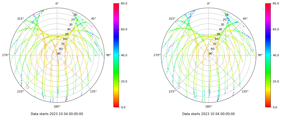
Skyplot for station CAAL. Parameter M1C Data file CAAL00ESP_R_2023277.xtr Skyplot for station CAAL. Parameter M2P Data file CAAL00ESP_R_2023277.xtr
