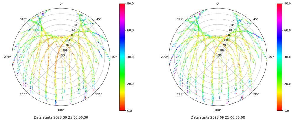
Skyplot for station CAAL. Parameter M1C Data file CAAL00ESP_R_2023268.xtr Skyplot for station CAAL. Parameter M2P Data file CAAL00ESP_R_2023268.xtr
