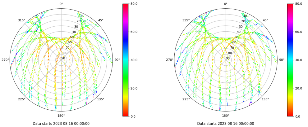
Skyplot for station CAAL. Parameter M1C Data file CAAL00ESP_R_2023228.xtr Skyplot for station CAAL. Parameter M2P Data file CAAL00ESP_R_2023228.xtr
